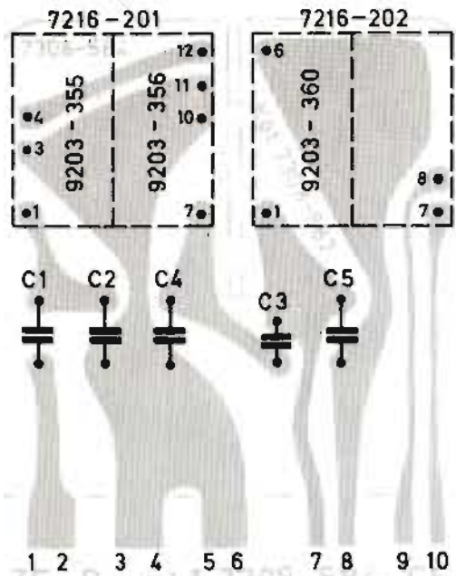
Filtre FI I, vu du côté des soudures
