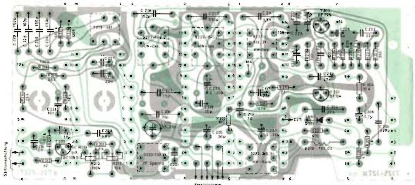
ZF-NF-Platte, Lötseite PLAQUETTE FI-BF, VUE DU COTE DES SOUDURES IF-AF Printed BOARD, SOLDER SIDE PIASTRA BF-FI, LATO SALDATURA
