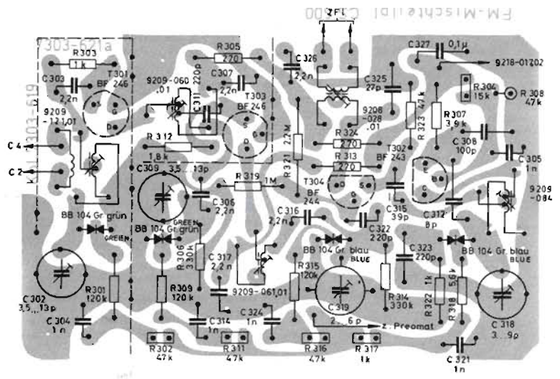
alties F-III Lötseite
