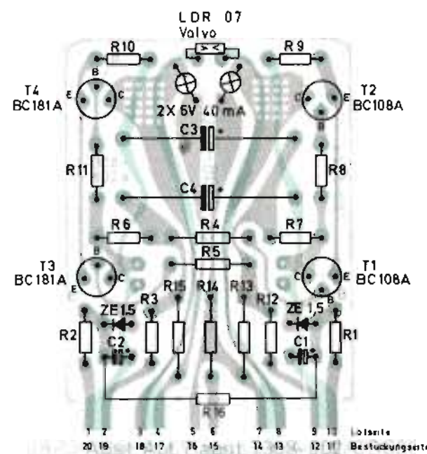
Plaquelette 56 V, vu du côté des soudures
