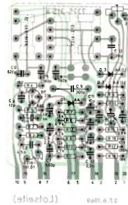
F VII Bestückungsseite F VII COMPONENT SIDE F VII VUE DU COTE DES COMPOSANTS F VII LATO COMPONENTI
