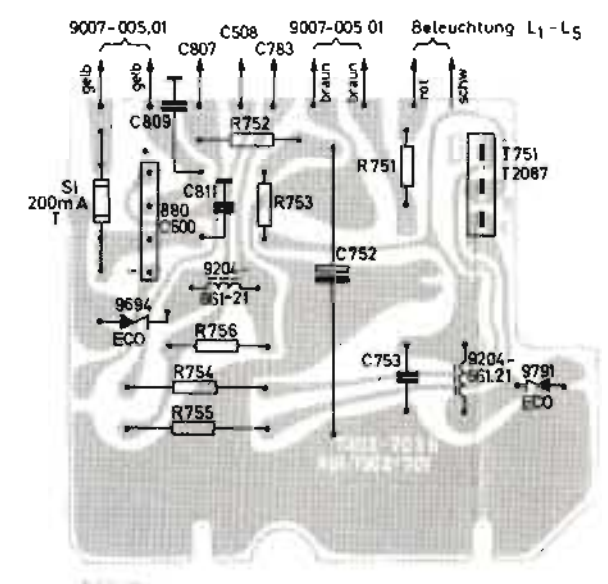
Bloc, vu du côté des composants
