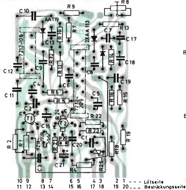
Plaquelette de connexion FM, vu du côté des soudures
