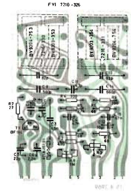
F VI Bestückungsseite F VI COMPONENT SIDE F VI VUE DU COTE DES COMPOSANTS F VI LATO COMPONENTI
