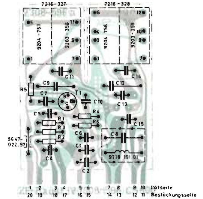
Filtre FI IV, vu du côté des soudures
