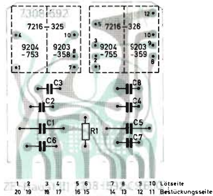
Filtre FI III, vu du côté des soudures
