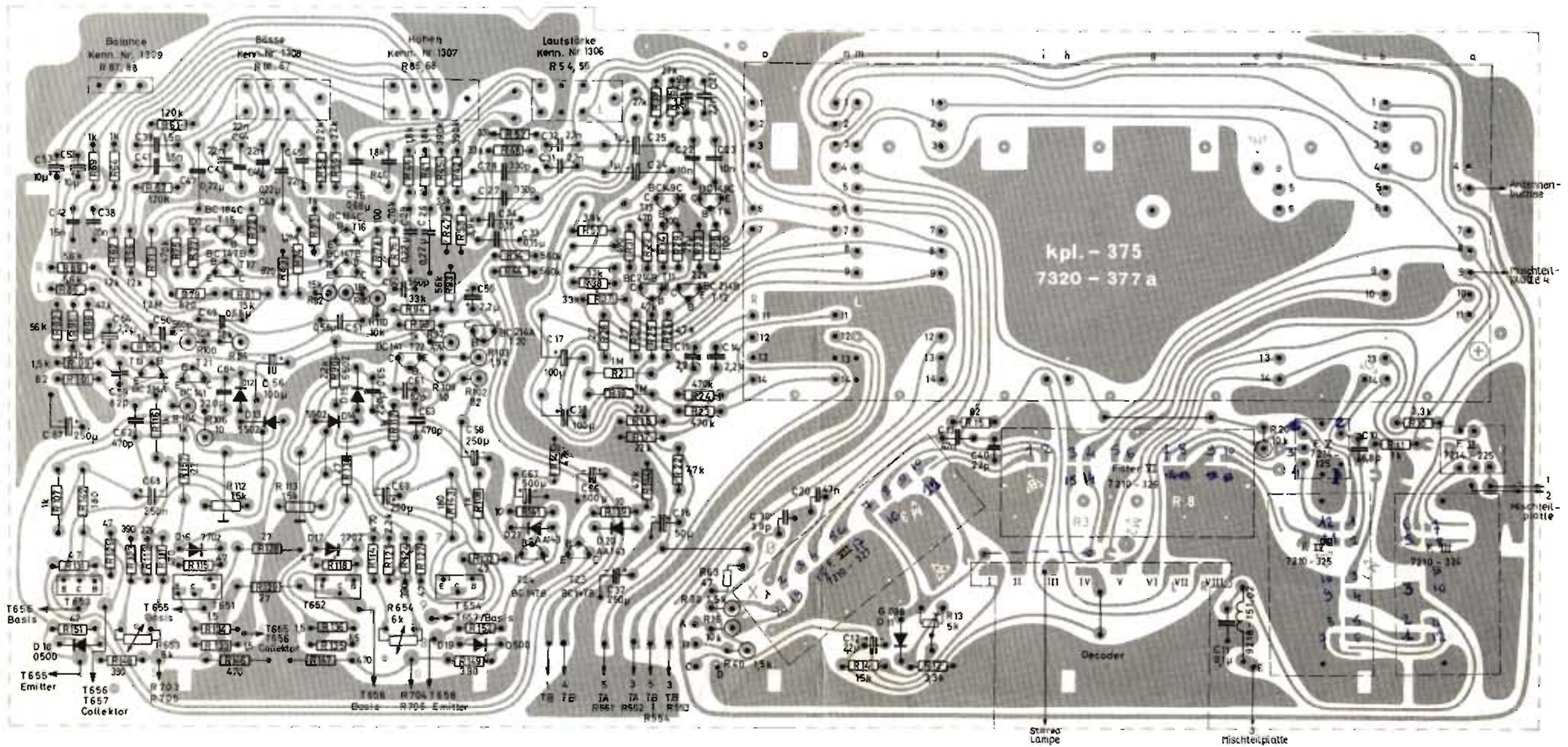
ZF-NF-Platte, Lötseite PLAQUETTE FI-BF, VUE DU COTE DES SOUDURES IF-AF Printed BOARD, SOLDER SIDE PIASTRA BF-FI, LATO SALDATURA
