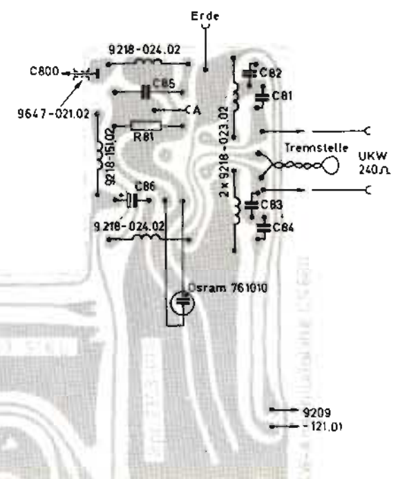
Bloc, vu du côté des composants
